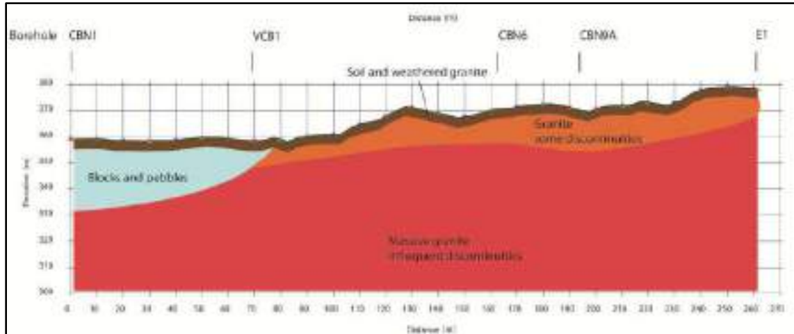
Figura 2-4. Perfil Geofísico P2.
