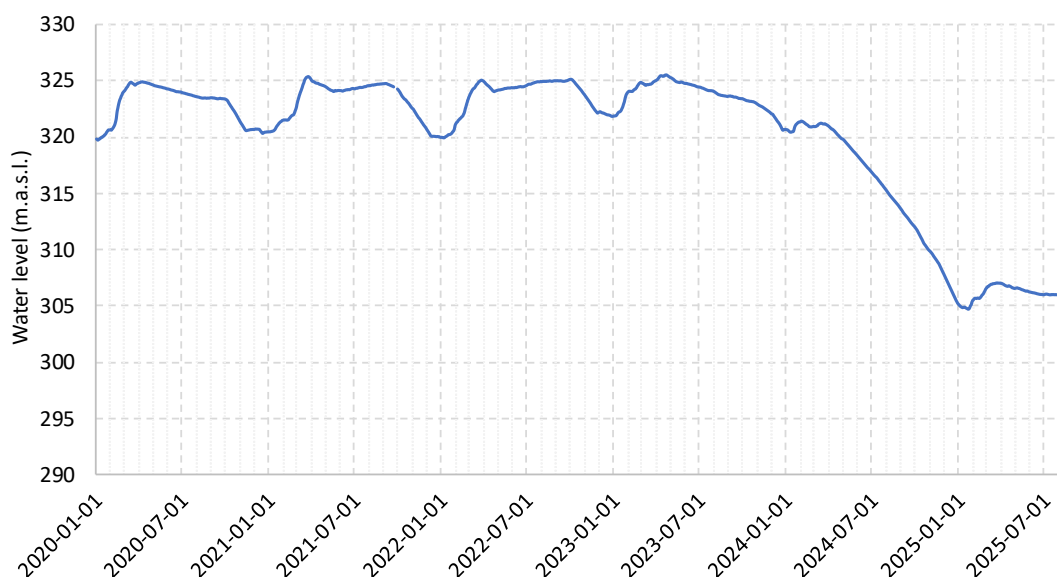
Figura 2-3 Medições diárias do nível da água na albufeira de Cahora Bassa (recebidas da HCB)
