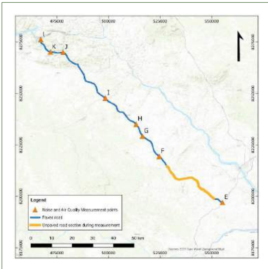
Figura 3 A Estrada N301 de 132 km entre a barragem e a N7.
