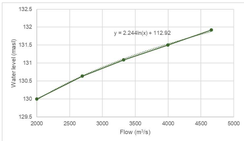
Figura 4-2. Fórmula interpolada para a relação entre o nível da água e o caudal no local proposto para a central hidroelétrica de Boroma.
