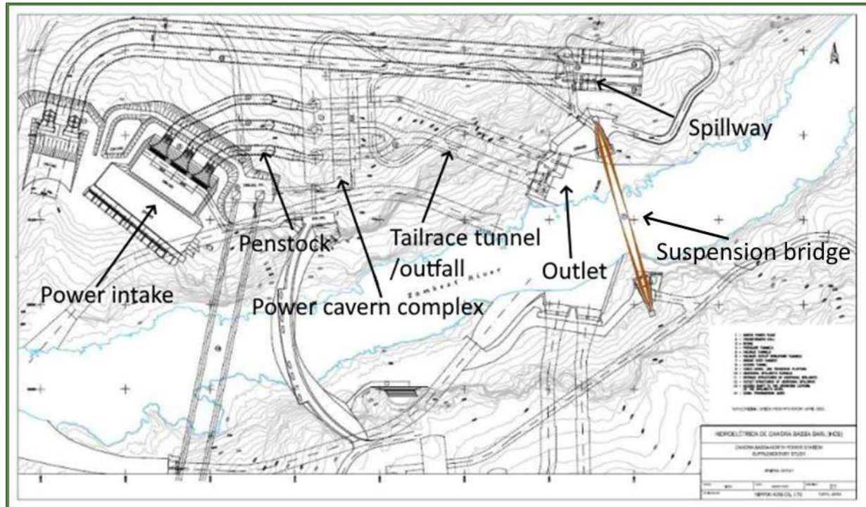
Figura 3-1: Disposição da Central hidroeléctrica da CBN
