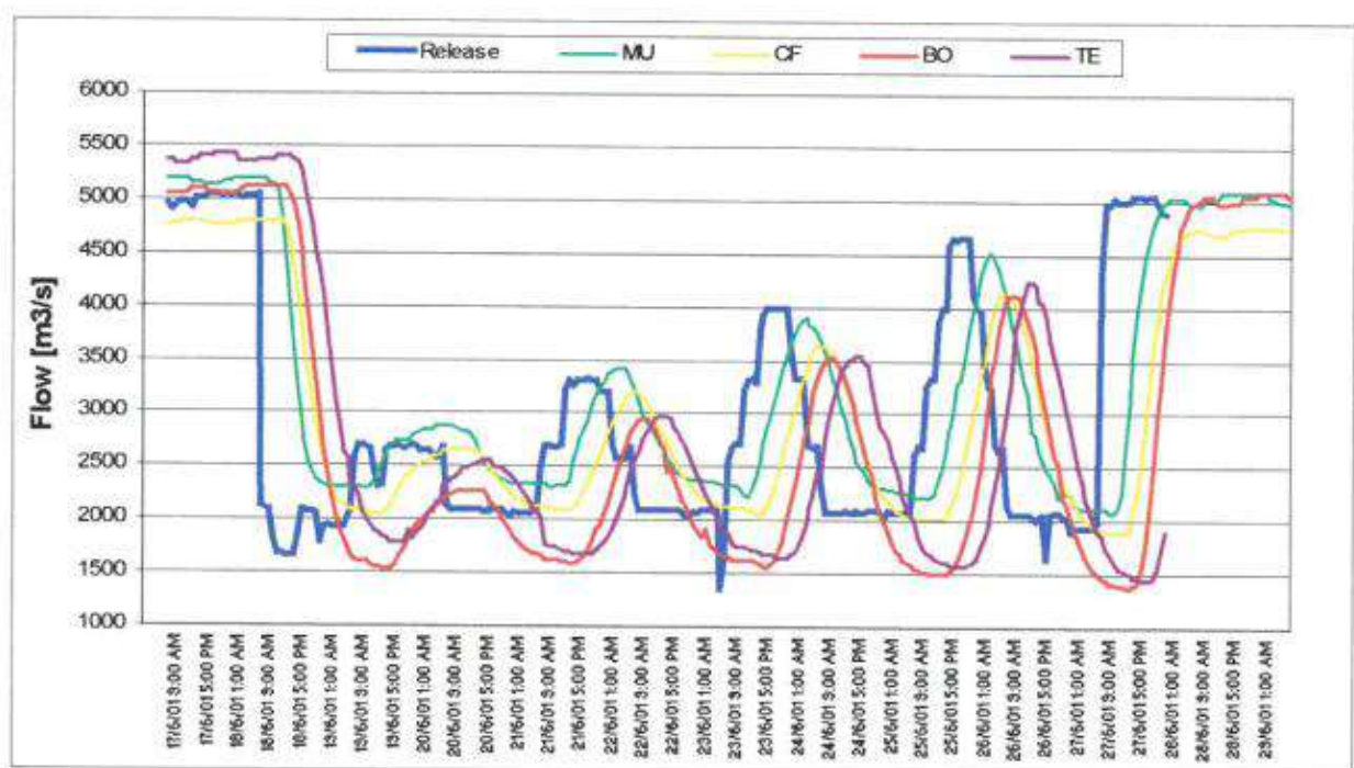
Figura 3-5. Segundo programa de testes de libertação de água de Cahora Bassa, Junho de 2001 – Caudais
