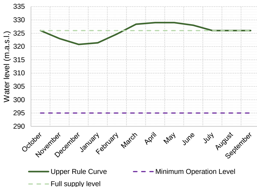
Figura 2-4 Curva de regra hidráulica operacional de Cahora Bassa
