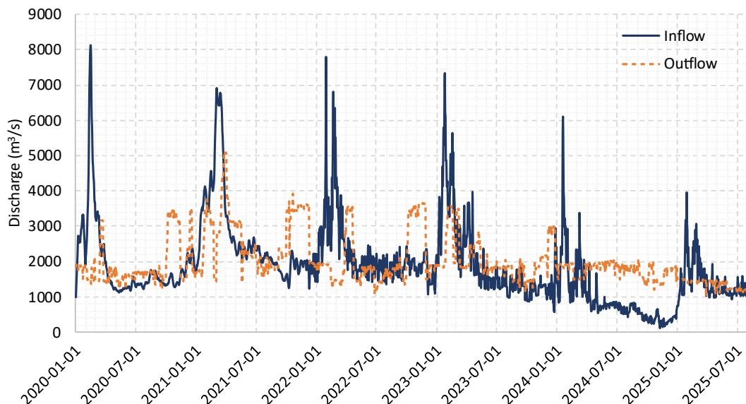
Figura 2-2 Medições diárias de entrada de água na albufeira de Cahora Bassa (recebidas da HCB).
