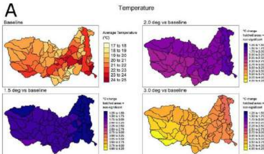
Figura 1 Alterações previstas na temperatura para três cenários de aquecimento global. Fonte: Hughes & Farinosi et al, 2020, Avaliando os impactos do desenvolvimento e da variabilidade climática nos recursos hídricos na bacia do Rio Zambezi. Simulando cenários futuros de clima e desenvolvimento.
