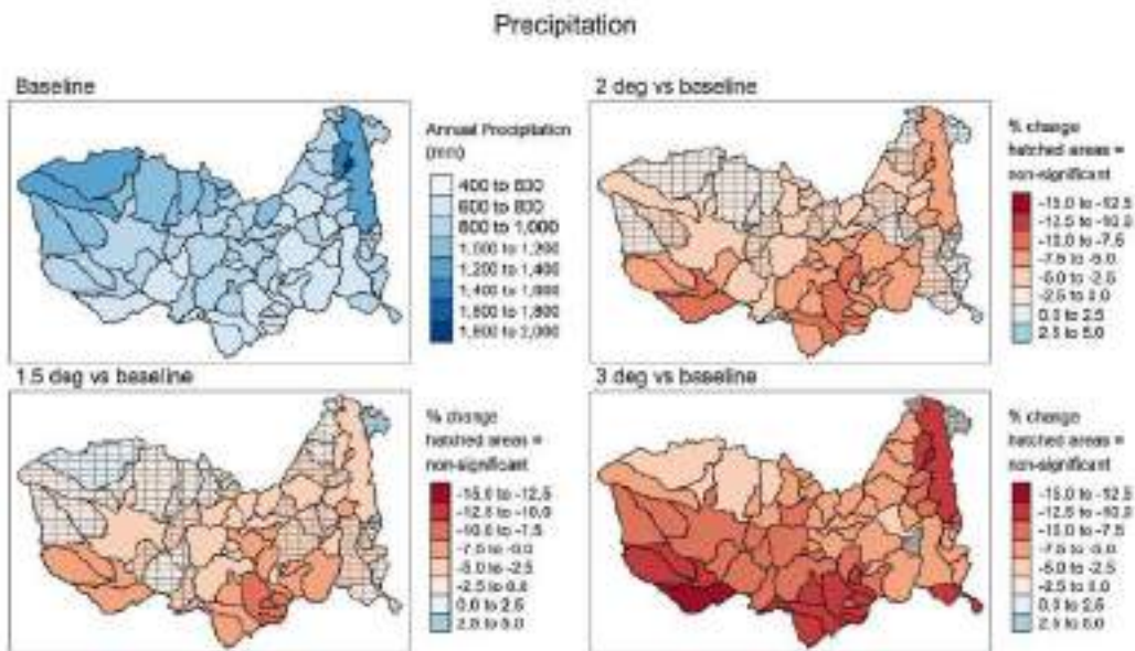
Figura 2 Alterações previstas na precipitação para três cenários de aquecimento global. Fonte: Hughes & Farinosi et al, 2020, Avaliando os impactos do desenvolvimento e da variabilidade climática nos recursos hídricos na bacia do Rio Zambezi. Simulando cenários futuros de clima e desenvolvimento
