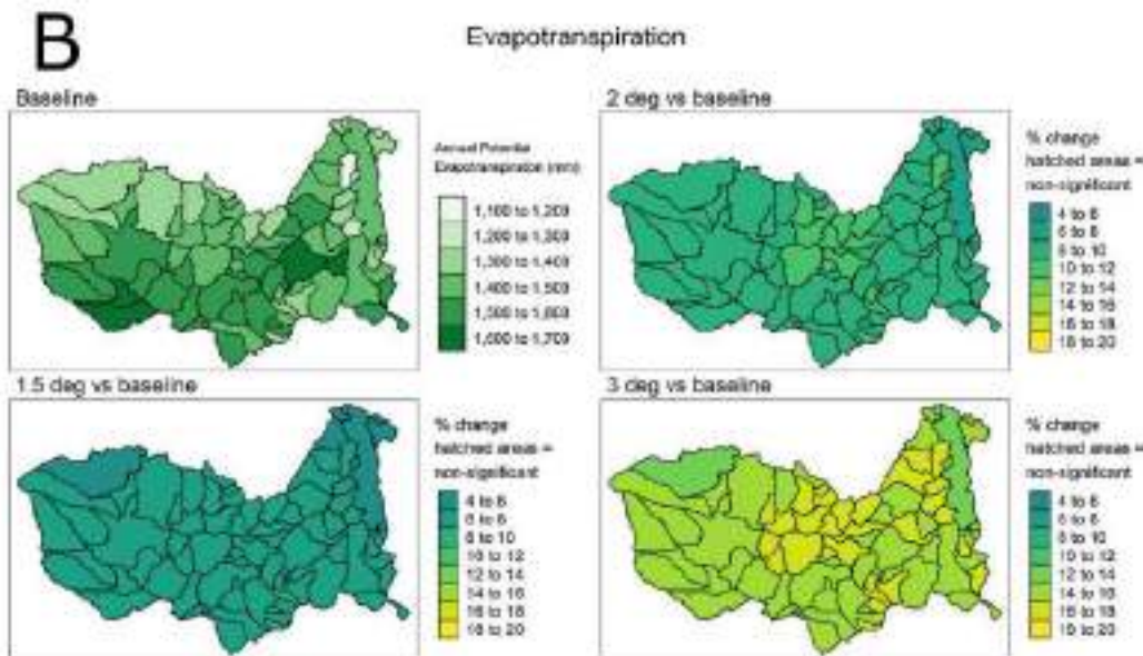
Figura 3 Alterações previstas na evapotranspiração para três cenários de aquecimento global. Fonte: Hughes & Farinosi et al, 2020, Avaliando os impactos do desenvolvimento e da variabilidade climática nos recursos hídricos na bacia do Rio Zambezi. Simulando cenários futuros de clima e desenvolvimento
