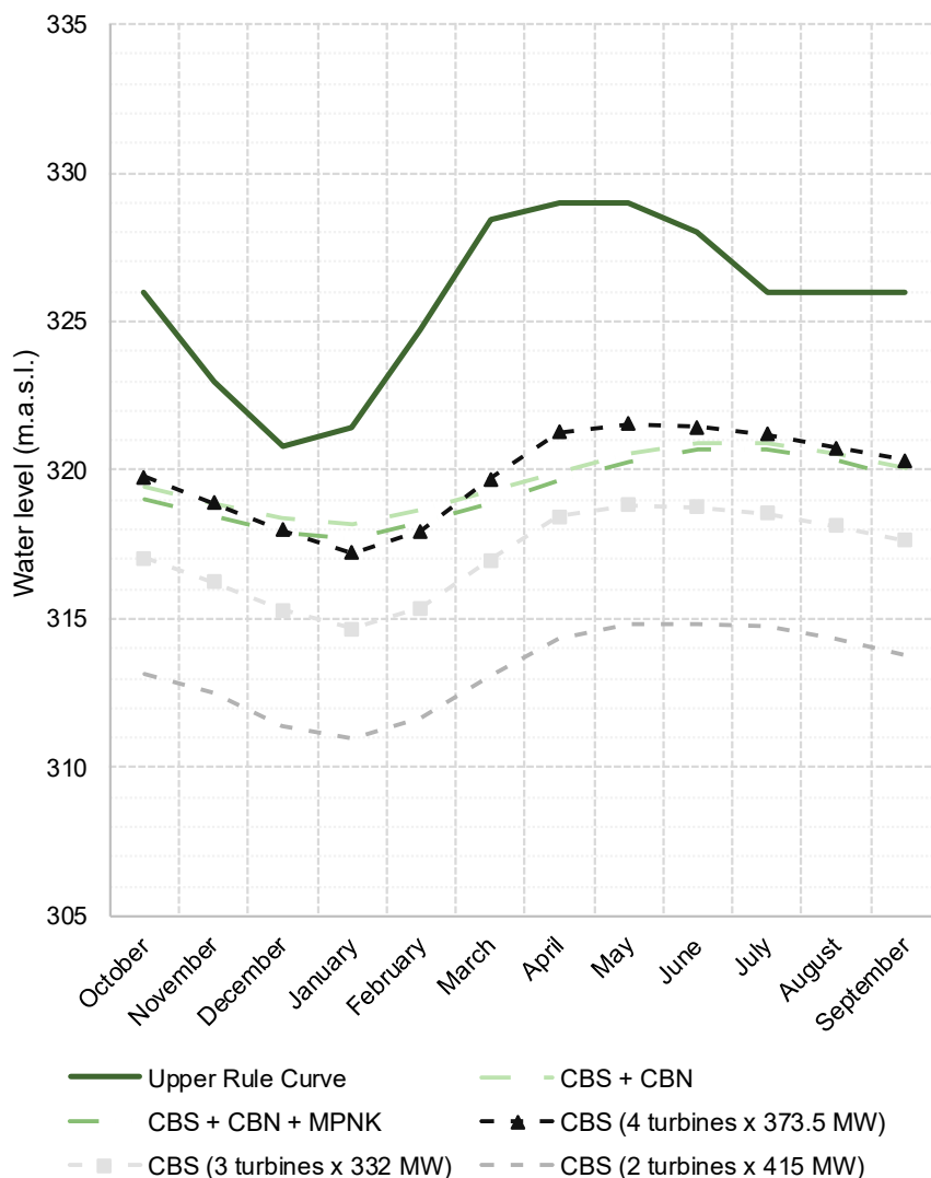
Figura 3-2 Curvas de operação recomendadas (superior e inferior) da albufeira de Cahora Bassa para CBS (actual), CBS+CBN e CBS+CBN+HMNK para diferentes cenários de operação.
