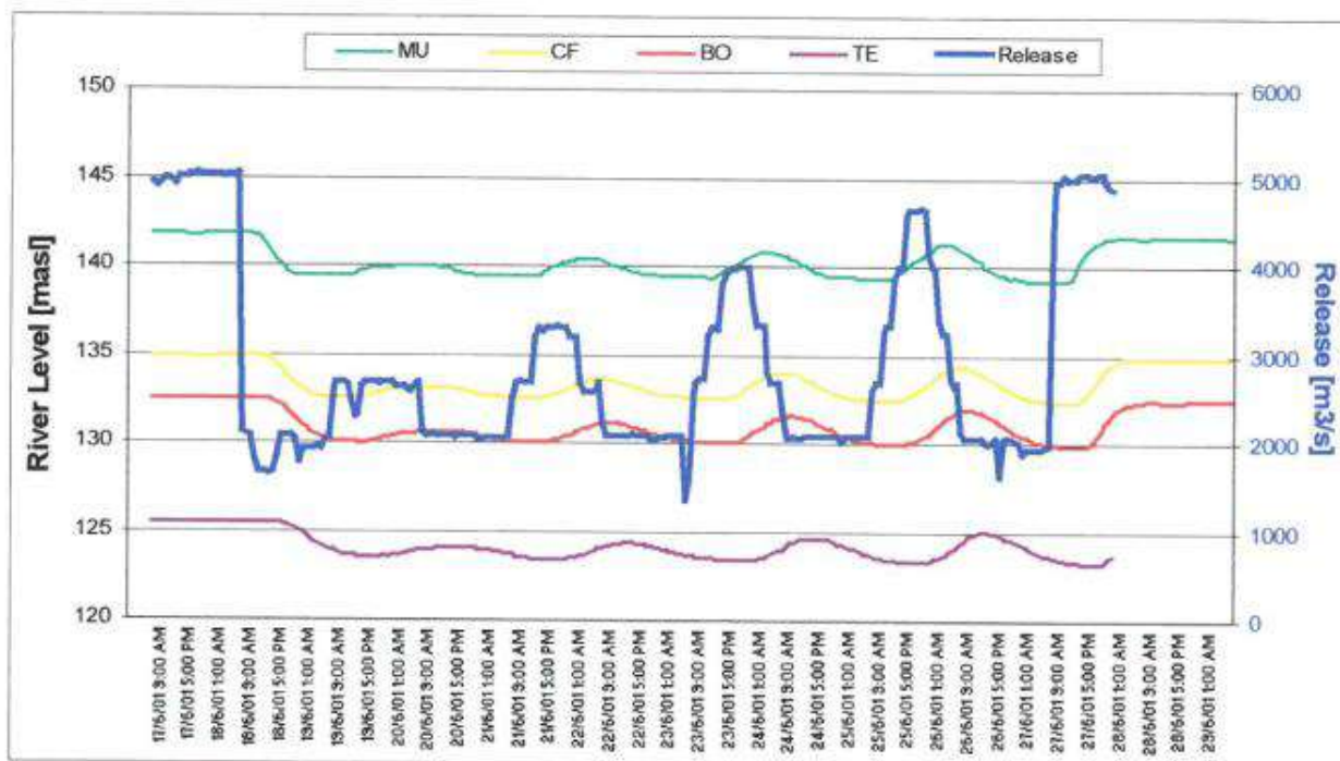
Figura 3-6. Segundo programa de testes de libertação de água de Cahora Bassa, Junho de 2001 – níveis da água.
