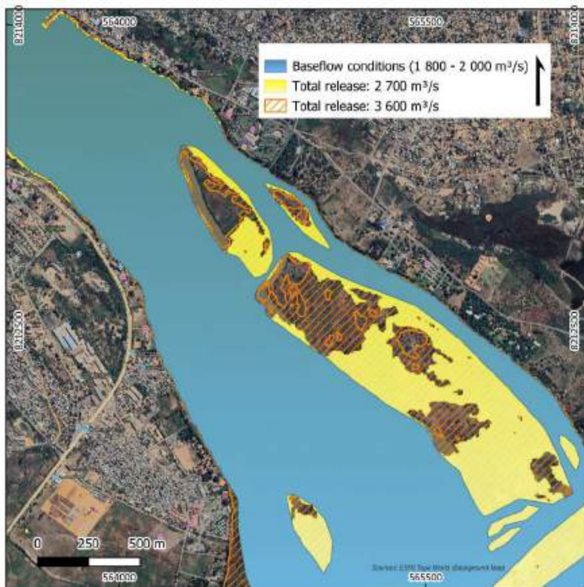
Figura 4-7. Impactos da subida do nível da água em Tete, a jusante da ponte, com os caudais mapeados a serem: 2.700 m³/s - adição de uma turbina da CBN com a CBS em pleno funcionamento e 3.600 m³/s - adição de três turbinas da CBN com a CBS em pleno funcionamento.
