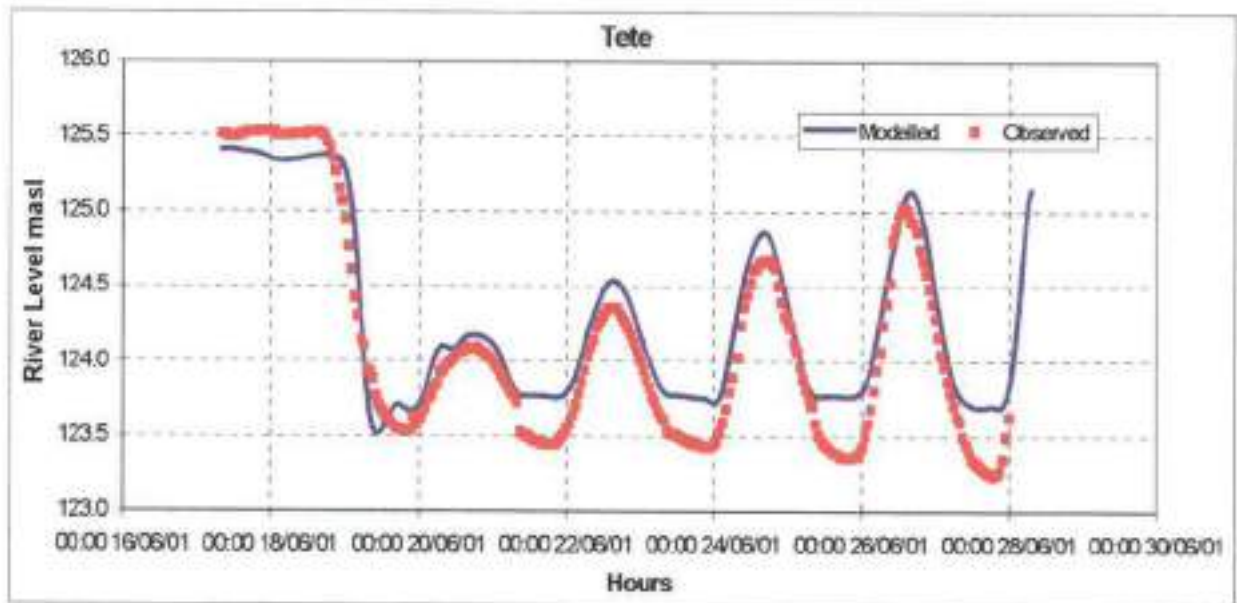
Figura 3-4. Segunda calibração do modelo de direccionamento de canais – Tete (Lahmeyer, 2001).
