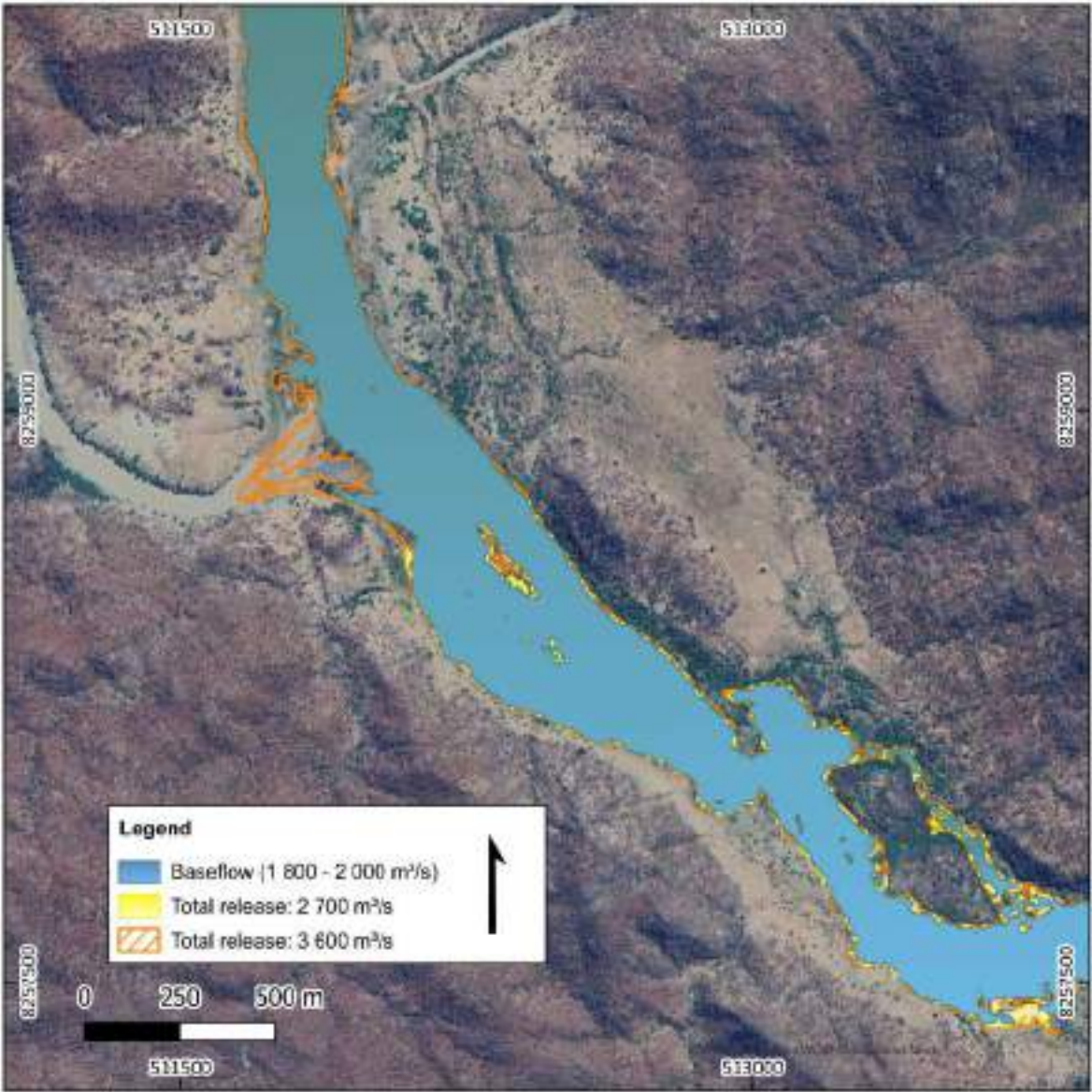
Figura 4-3 Impactos da subida do nível da água no local proposto para a barragem de Mphanda Nkuwa: os caudais mapeados são: 2.700 m³/s - adição de uma turbina da CBN com a CBS em pleno funcionamento e 3.600 m³/s - adição de três turbinas da CBN com a CBS em pleno funcionamento.
