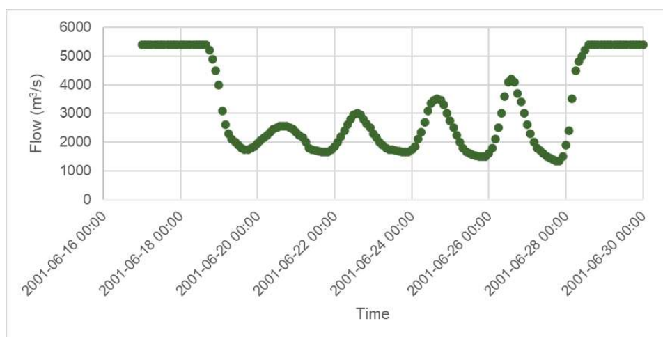
Figura 4-9. Séries temporais de entrada para o modelo Mike+, que é uma réplica da série de caudais de Lahmeyer.
