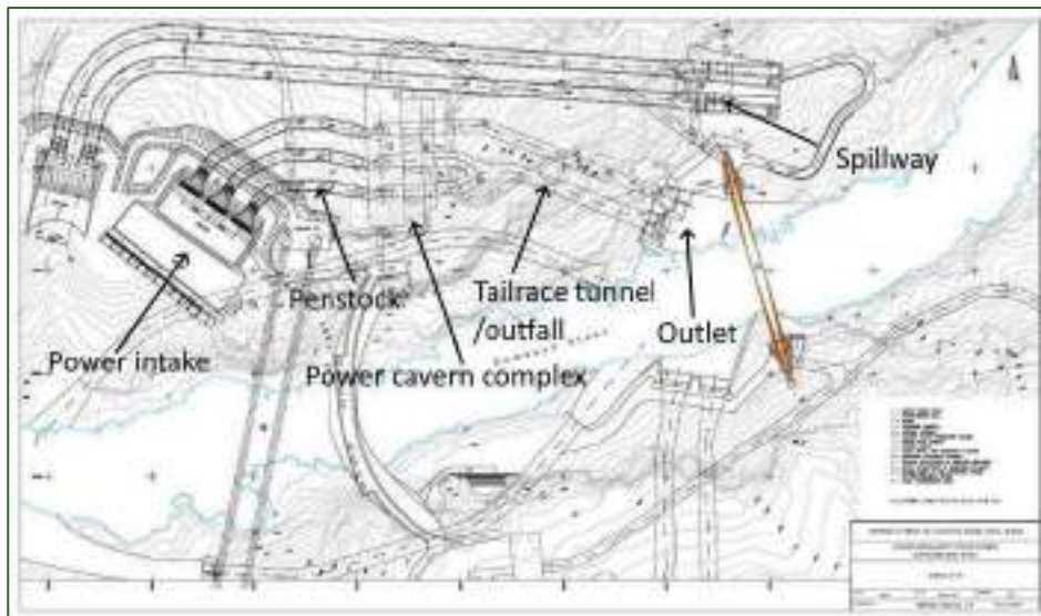
Figura 4: Disposição da Central Hidroeléctrica CBN
