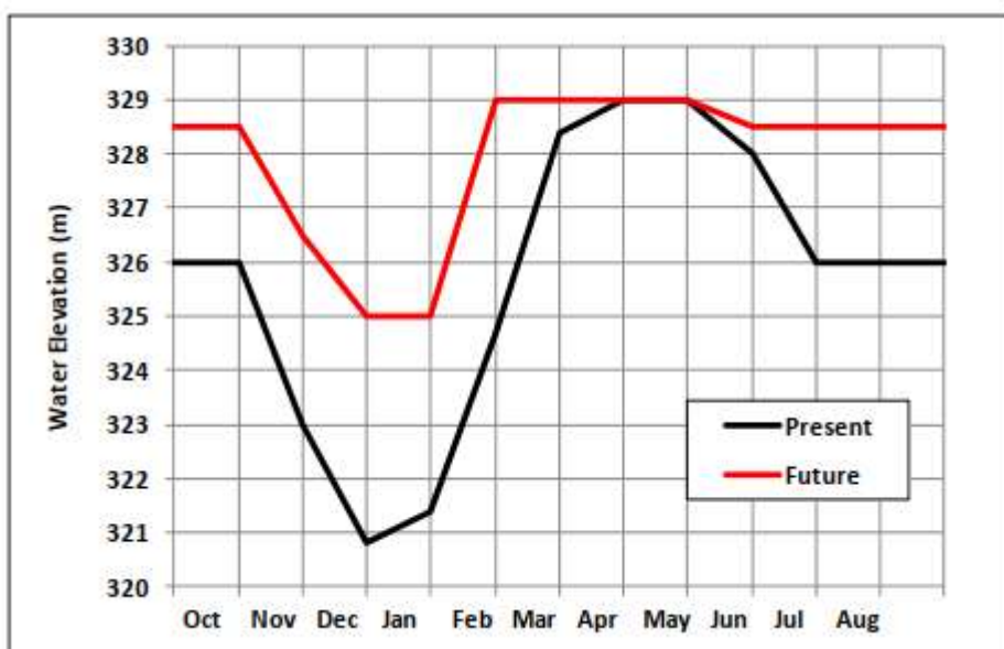
Figura 3-1 Curva preliminar de operação da albufeira de Cahora Bassa com CBN (Nippon Koei UK, 2013).
