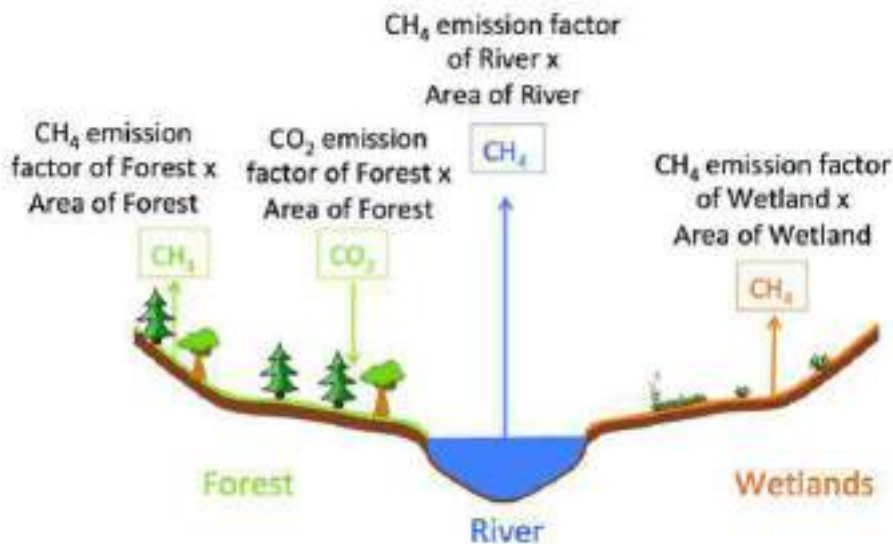
Figura 4 Esquema de um exemplo de paisagem pré-represa como um mosaico de áreas ecológicas com diferentes comportamentos de GEE. Fonte: Mercier-Blais et al. 2020. Avaliação da pegada líquida de gases de efeito estufa para a albufeira de Cahora Bassa (Moçambique) usando o método da ferramenta G-res, Reservoir G-res # 2.102045, G-res Tool v2.1
