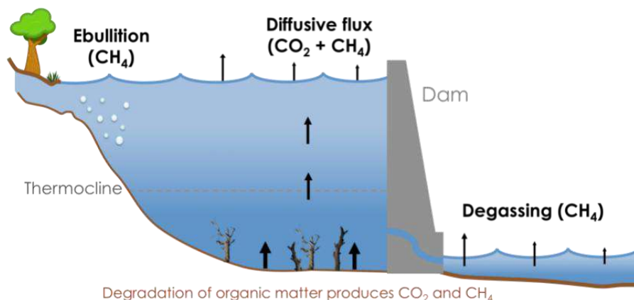
Figura 5 Esquema das quatro vias de emissão de GEE no G-res: emissões difusivas de CO 2 , emissões difusivas de CH 4 , emissões borbulhantes de CH 4 e emissões de degaseificação de CH 4 . Fonte: Mercier-Blais et al. 2020. Avaliação da pegada líquida de gases de efeito estufa para a albufeira de Cahora Bassa (Moçambique) usando o método da ferramenta G-res, Albufeira G-res # 2.102045, Ferramenta G-res v2.1
